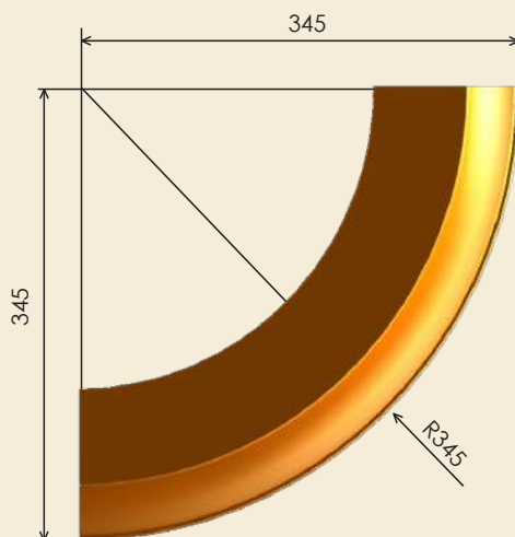
Профіль зовнішнього карниза №4
