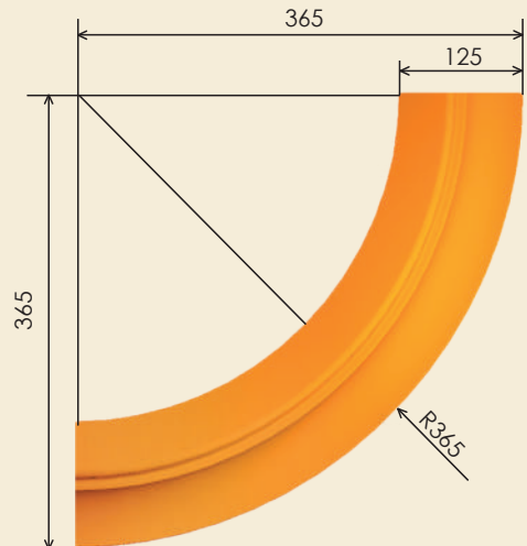
Профіль зовнішнього карниза №2
