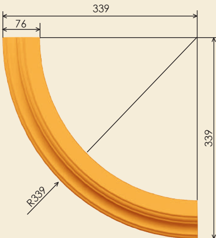
Профіль зовнішнього карниза №1
