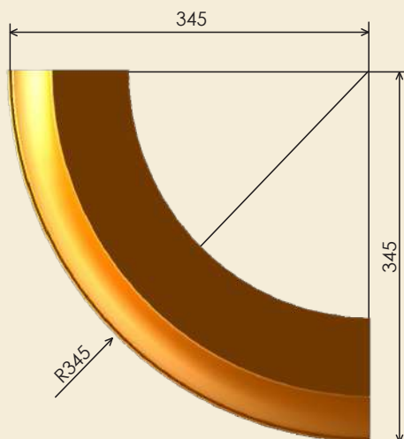
Профіль зовнішнього карниза №5
