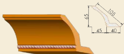
Карниз прямий №5 Довжина 2000 та 2500 мм
