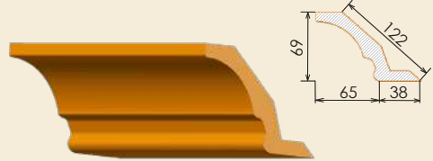
Карниз прямий №2 Довжина 2000 та 2500 мм
