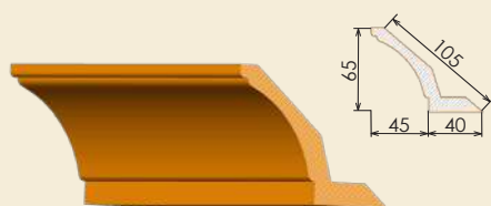
Карниз прямий №4 Довжина 2000 та 2500 мм
