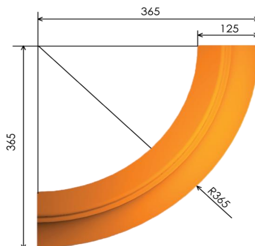
Профіль наружного карнизу №2
