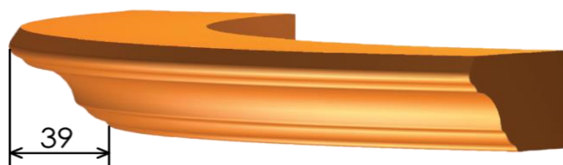
Карниз верхній прямий №1
