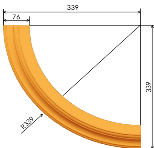
Профіль наружного карнизу №1
